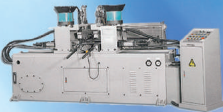
▶ Y-2000 全自動入螺母套及縮管機
