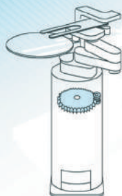
機械手臂的旋轉機構
