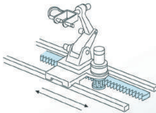
長行程工作機械
