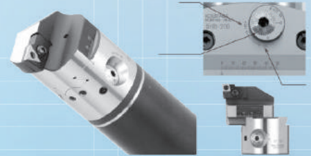
ABH 精塘孔頭
