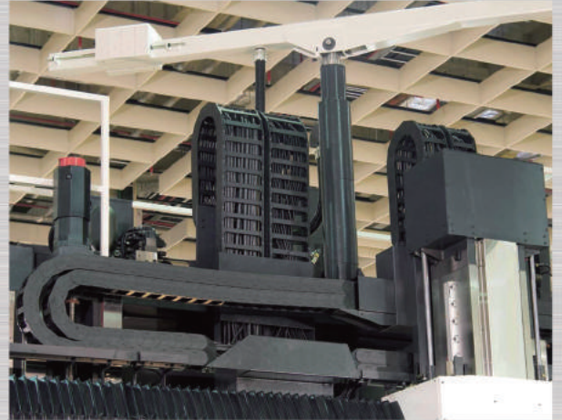
鏈條護管 (工程塑鋼)
