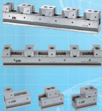
SVF 彈性化並列式虎鉗
