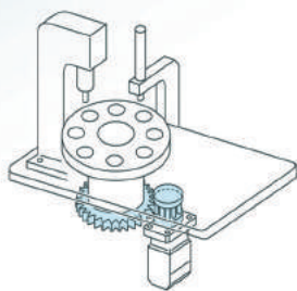
分度旋轉台
