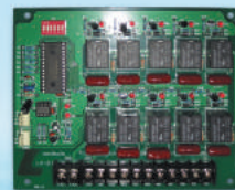
脈衝控制儀
