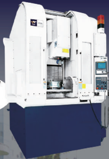
立式 QVM-610AW 臥式 MA-24AW 鋁合金鋼圈鑽孔機
