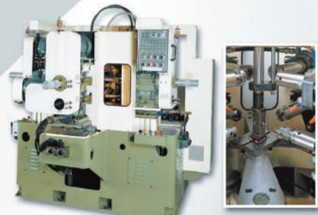
八軸油壓自動加工專用機床
