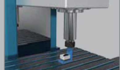
Perpendicularity主軸垂直度
