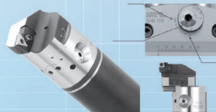
ABH 精塘孔頭
