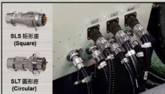
電子電源接頭 (UL認證編號:E313914)
