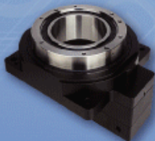
中空旋轉平台 YZMR60-300 Series
